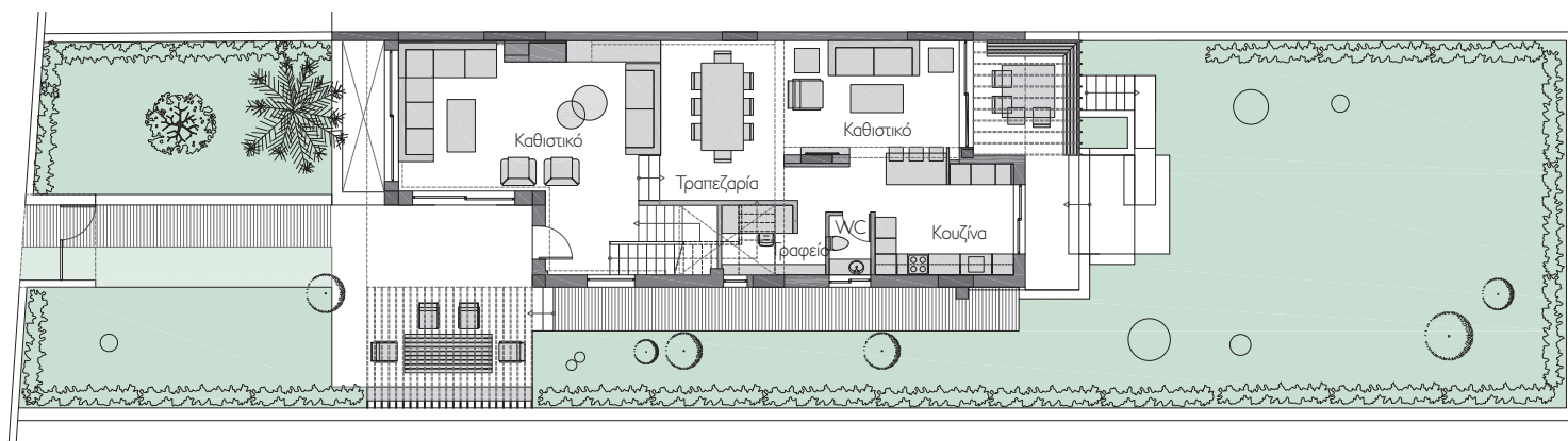
ΚΑΤΩΦΗ ΙΣΟΓΕΙΟΥ
